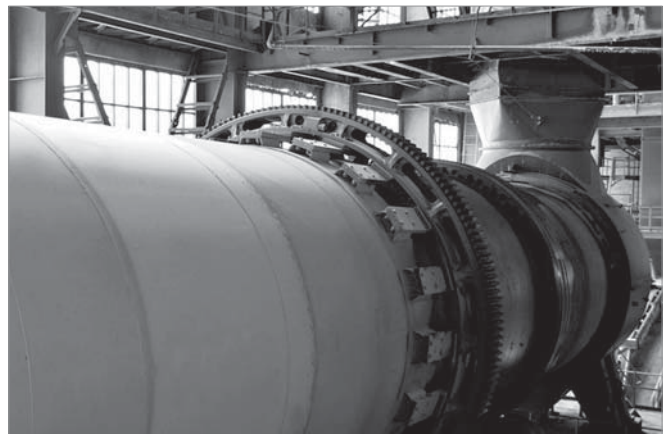
Барабан-гранулятор. Виробництво вапняково-аміачної селітри
